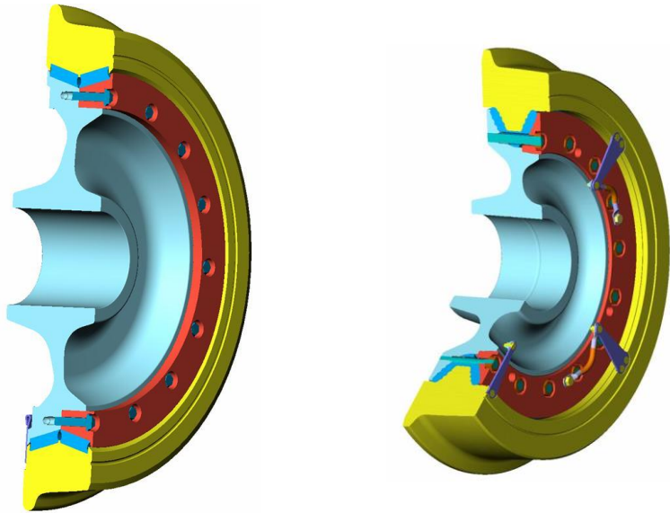
GHH®V15 / GHH®V30
